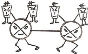
ISOMÈRE BIMÈRE "La ronde des enfants" 2 H 2 O
