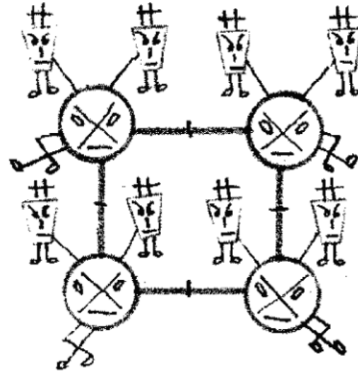
ISOMÈRE QUADRIMÈRE "L'enclos fermé" 4 H 2 O
