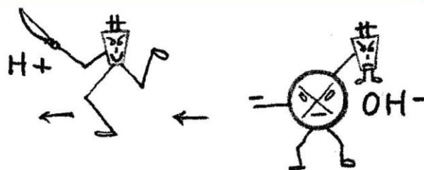
L'IONISATION DE H 2 O
