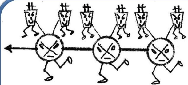
ISOMÈRE TRIMÈRE "Le petit train grande vitesse" 3 H 2 O
